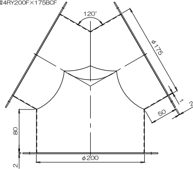
質量 1788g フランジ付異径Y管4RY200F×175BCF
