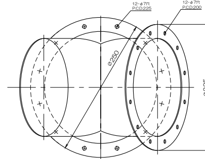
質量 1536g フランジ付異径Y管4RY200F×175(B)CF
