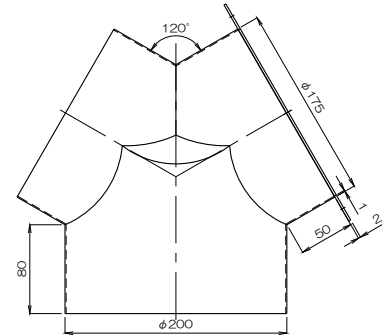
質量 1252g フランジ付異径Y管4RY200×175(B)CF
