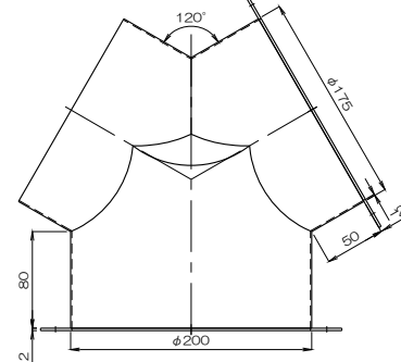
質量 1536g フランジ付異径Y管4RY200F×175(B)CF
