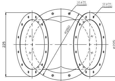
質量 1788g フランジ付異径Y管4RY200F×175BCF
