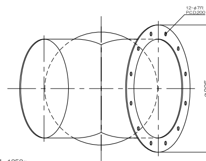
質量 1252g フランジ付異径Y管4RY200×175(B)CF
