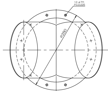
質量 1284g フランジ付異径Y管4RY200F×175BCF
