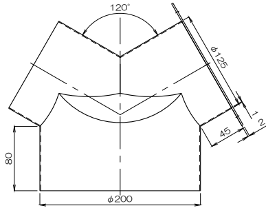
質量 1127g フランジ付異径Y管4RY200×125IB/CF
