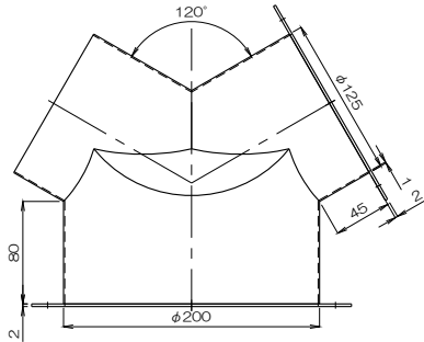
質量 1411g フランジ付異径Y管4RY200F×125IB/CF
