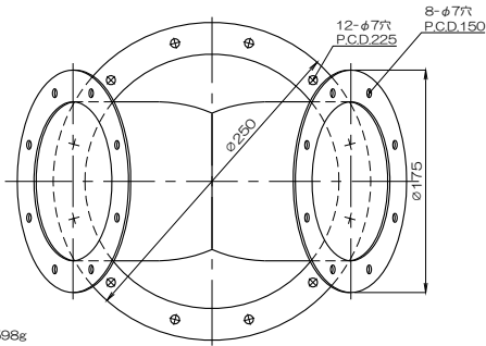
質量 1598g フランジ付異径Y管4RY200F×125BCF
