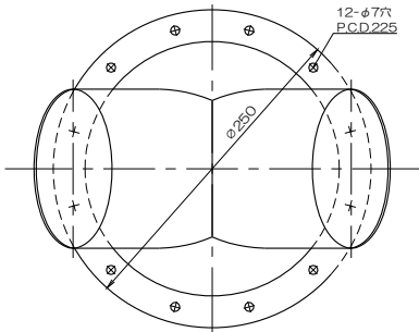
質量 1224g フランジ付異径Y管4RY200F×125
