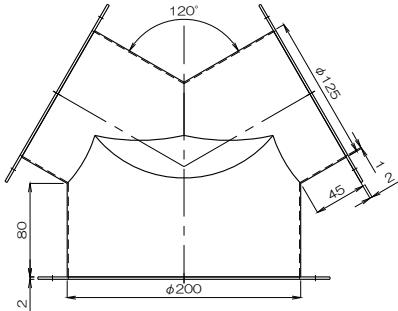
質量 1598g フランジ付異径Y管4RY200F×125BCF
