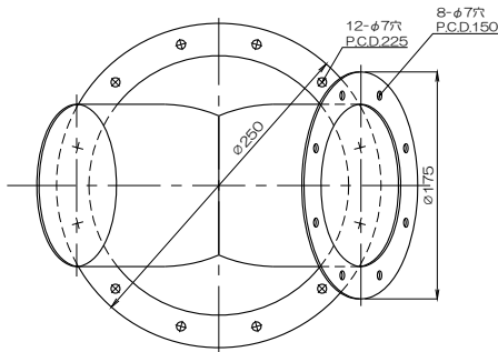
質量 1411g フランジ付異径Y管4RY200F×125IB/CF
