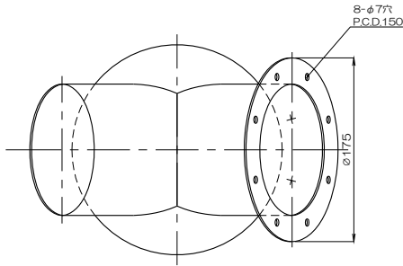
質量 1127g フランジ付異径Y管4RY200×125IB/CF
