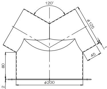
質量 1224g フランジ付異径Y管4RY200F×125
