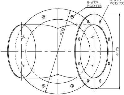
質量 1047g フランジ付異径Y管4RY150F×125(B)CF
