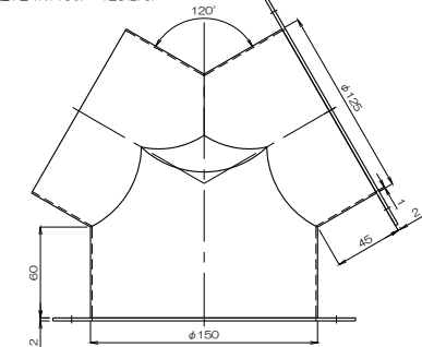
質量 1047g フランジ付異径Y管4RY150F×125(B)CF
