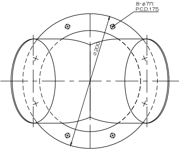
質量 860g フランジ付異径Y管4RY125F×125
