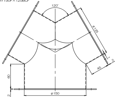
質量 1234g フランジ付異径Y管4RY150F×125BCF
