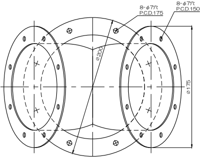
質量 1234g フランジ付異径Y管4RY150F×125BCF
