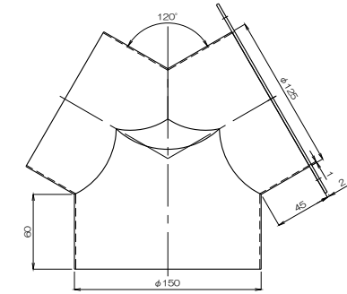
質量 827g フランジ付異径Y管4RY150×125(B)CF
