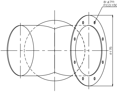
質量 827g フランジ付異径Y管4RY150×125(B)CF
