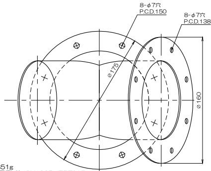
質量 851g フランジ付異径Y管4RY100F×75(B)CF
