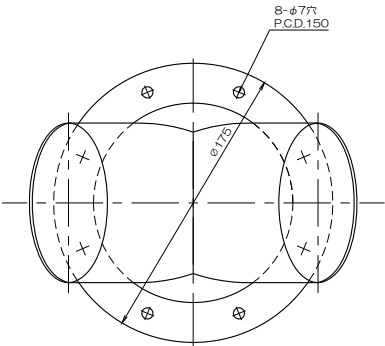
質量 657g フランジ付異径Y管4RY125F×100
