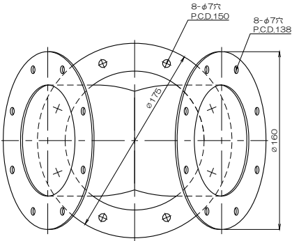
質量 1045g フランジ付異径Y管4RY125F×100BCF
