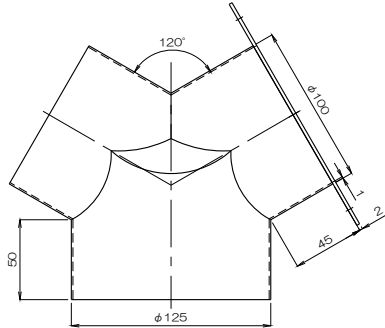
質量 664g フランジ付異径Y管4RY125×100(B)CF
