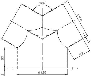
質量 657g フランジ付異径Y管4RY125F×100
