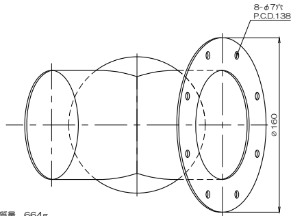
質量 664g フランジ付異径Y管4RY125×100(B)CF
