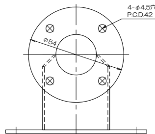
質量 195g フランジ付異径T管4RT38F×25BCF
