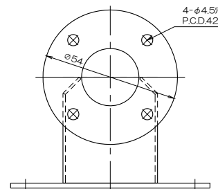
質量 166g フランジ付異径T管4RT38F×25B(C)F
