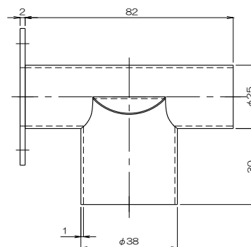
質量 104g フランジ付異径T管4RT38×25B(C)F
