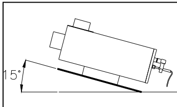
ホットスタート運転での取付姿勢 (XS-2シリーズ A・Bセンサ付、XS-4・5・6シリーズ)
