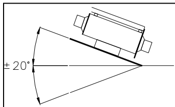
通常運転での取付姿勢 400℃以上で使用する場合
