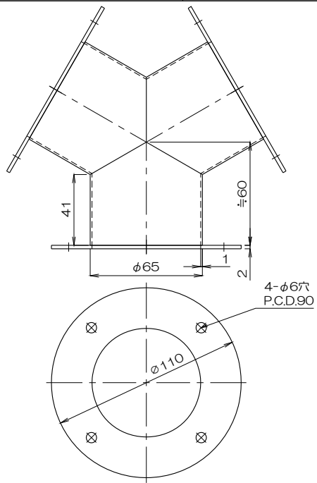
質量 507g フランジ付Y管 4Y 65ABCF
