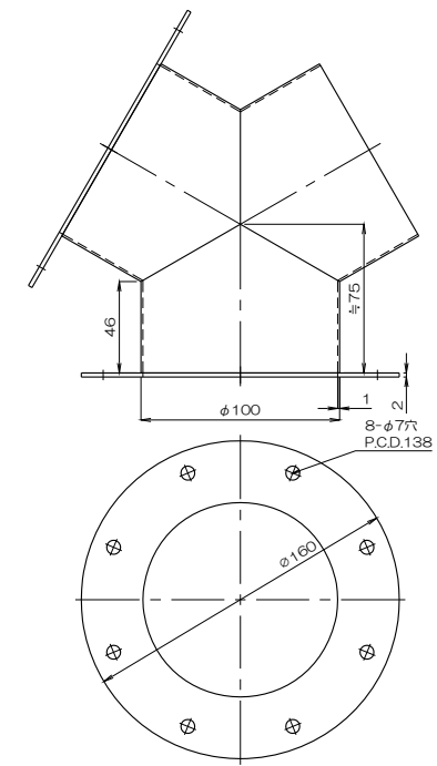
質量 574g フランジ付Y管 4Y 100A(B,C)F
