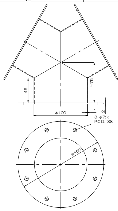
質量 962g フランジ付Y管 4Y 100ABCF
