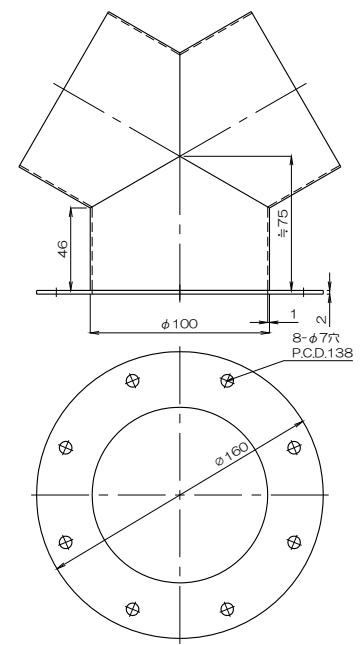
質量 574g フランジ付Y管 4Y 100A(B,C)F
