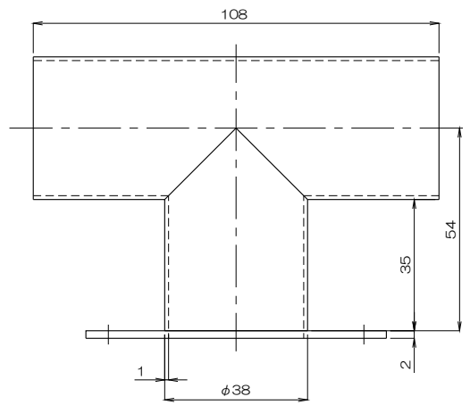
質量 182g フランジ付T管4T38 AF
