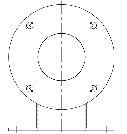
質量 244g フランジ付T管4T38 AB(C)F
