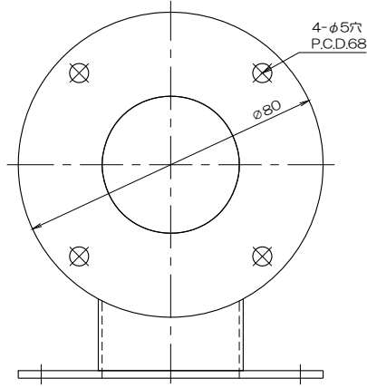
質量 306g フランジ付T管4T38 ABCF
