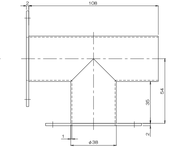
質量 182g フランジ付T管4T38 B(C)F
