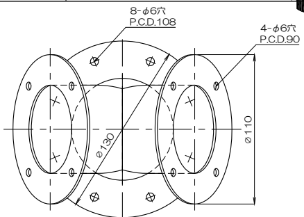
質量 558g フランジ付異径Y管4RY75F×65BCF
