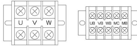
ネジサイズ M6
