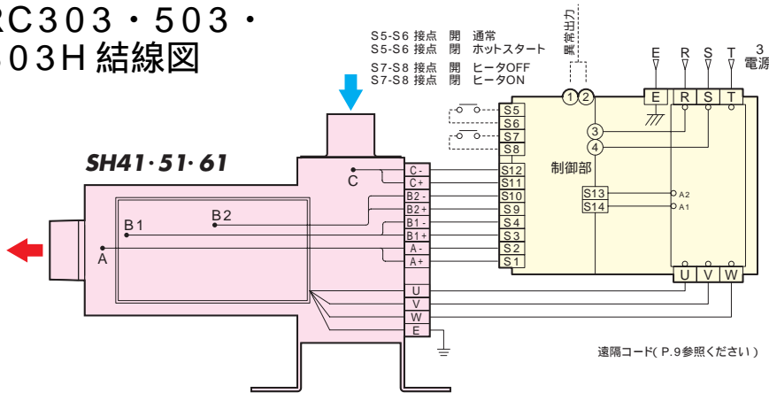
TRC803・ 503H 結線図
