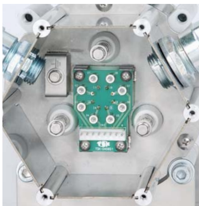
SH41・51・61 配線接続部(A視)
