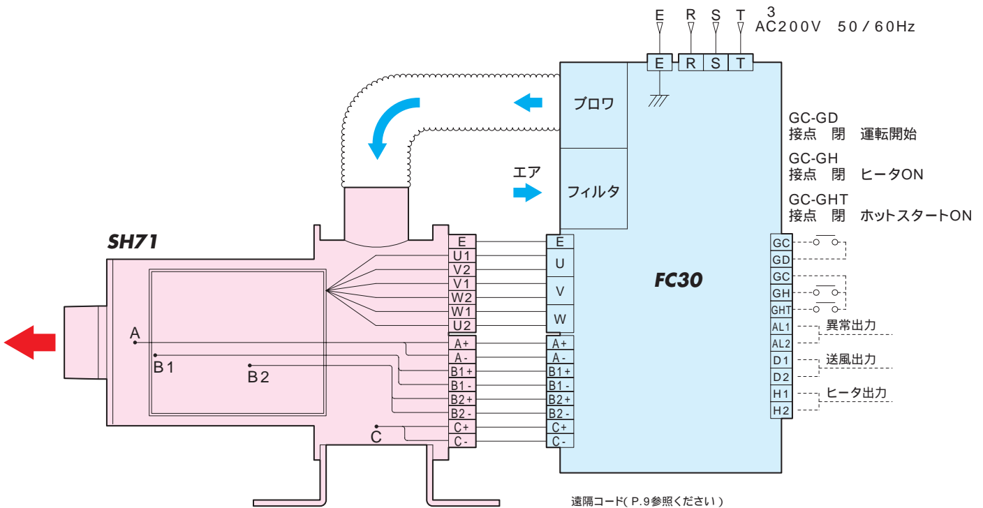
SH71 結線図 (FC30)
