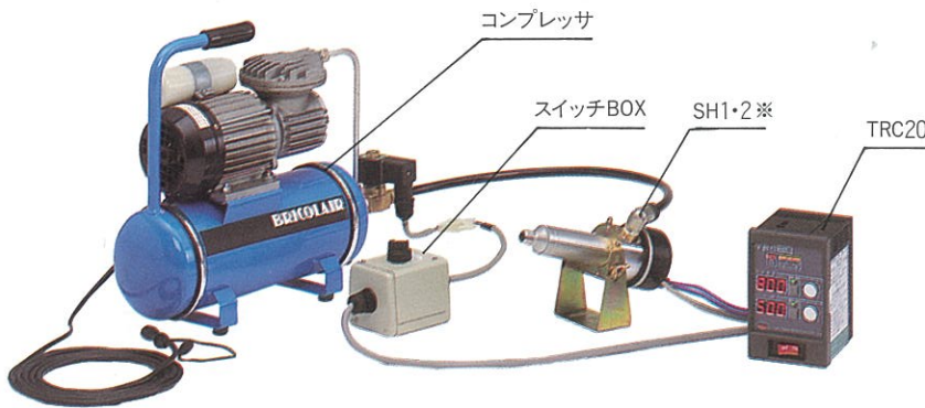
※OP. φ12ワンタッチホースジョイント付
