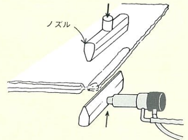
マシン掛の前のカセン毛布の熱風接着に プレスに取り付けノズルを上下させる
