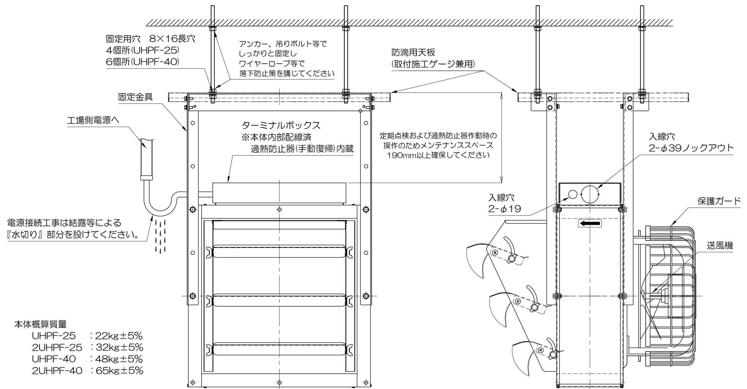
UHPF吊り下げ施工図
