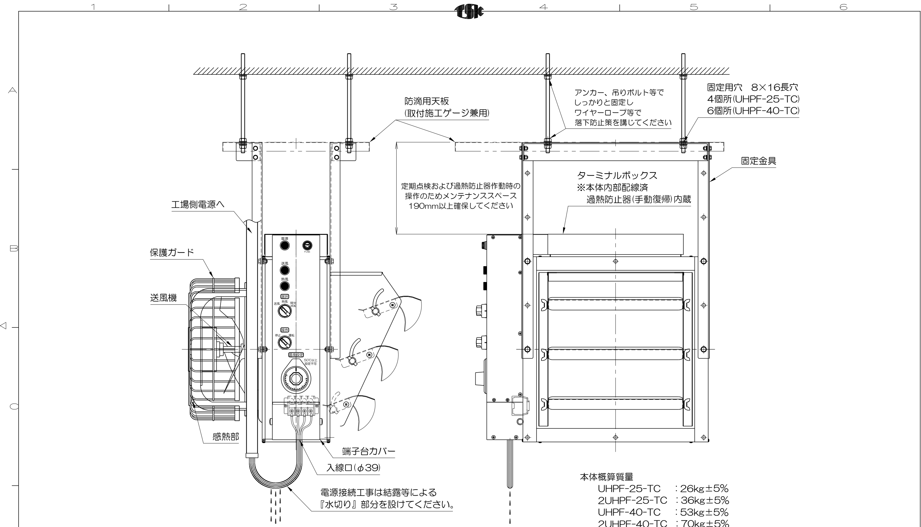
UHPF-TC吊り下げ施工図
